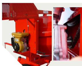
Entraînement pignon chaîne sur modèle 430 l.
